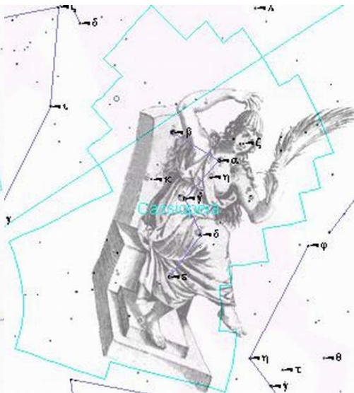
Созвездие Кассиопея
